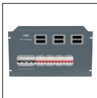
DISTRIBUTORE 125A IN: 1x125A 3P+N+T CEE OUT: 4x63A 3P+N+T CEE
