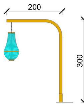
SUPPORTO A SBALZO - CANTILEVER SUPPORT
