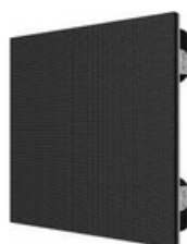
LED WALL PASSO 2.5 INDOOR SERIE ABSEN POLARIS Mattonelle: 50x50 cm Accessori: - Flying bar 50 cm per sospensione - Sending card NovaStar MCTRL 4K
